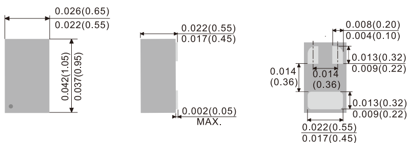
DFN 3L
