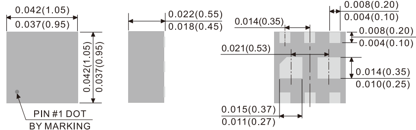
DFN1010-6L
