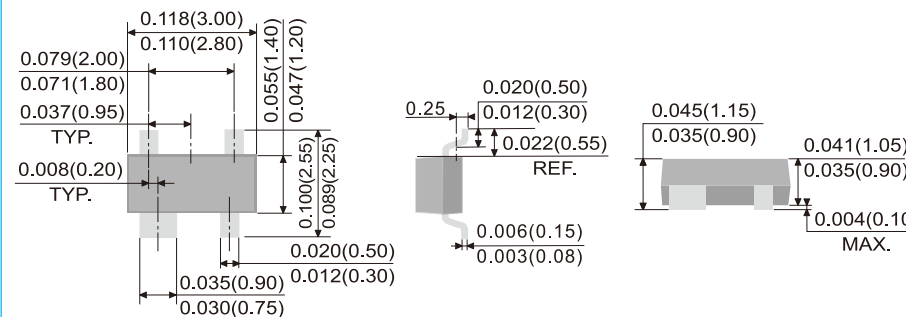
SOT-143
