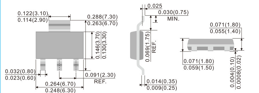
SOT-223
