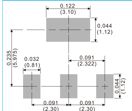
SOT-89
