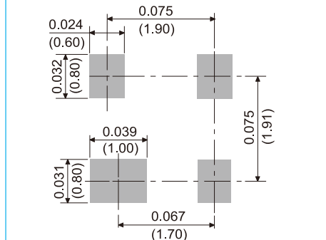
SOT-143
