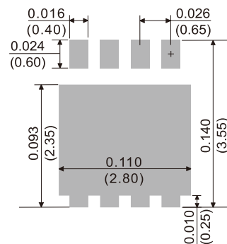
DFN3333-8L
